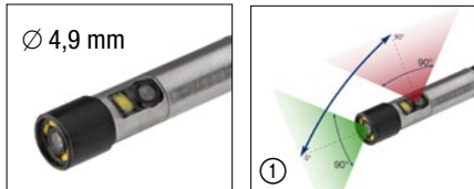
Caméra frontale et latérale
