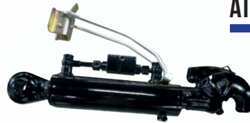
400€HT 320€HT BARRE DE POUSSÉE HYDRAULIQUE Rotule Cat 2 et Crochet Cat 3 Tige de 36 mm - Piston de 70 mm Longueur Mini 600 Longueur Maxi 810 N°269
